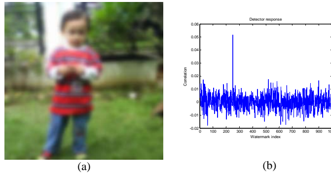
Fig. 14. Image blurring
